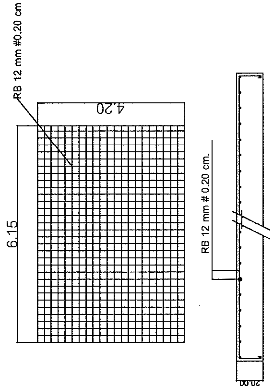
ฐานเครื่องกำเนิดไฟฟ้า
